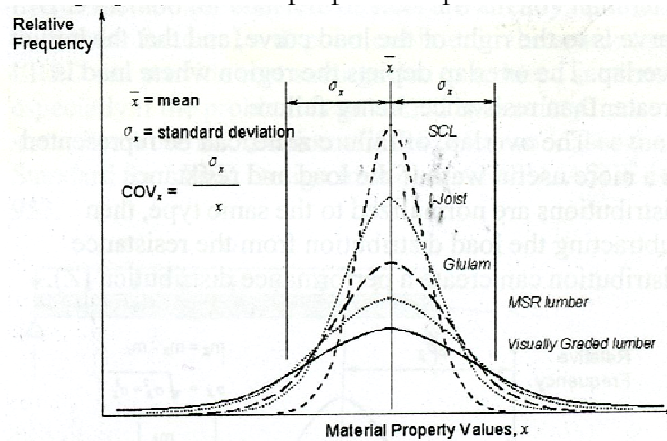
Figura 1.2. Representación de la variabilidad de una propiedad estructural para varios productos de madera (Adaptado de Taylor, 2001)
