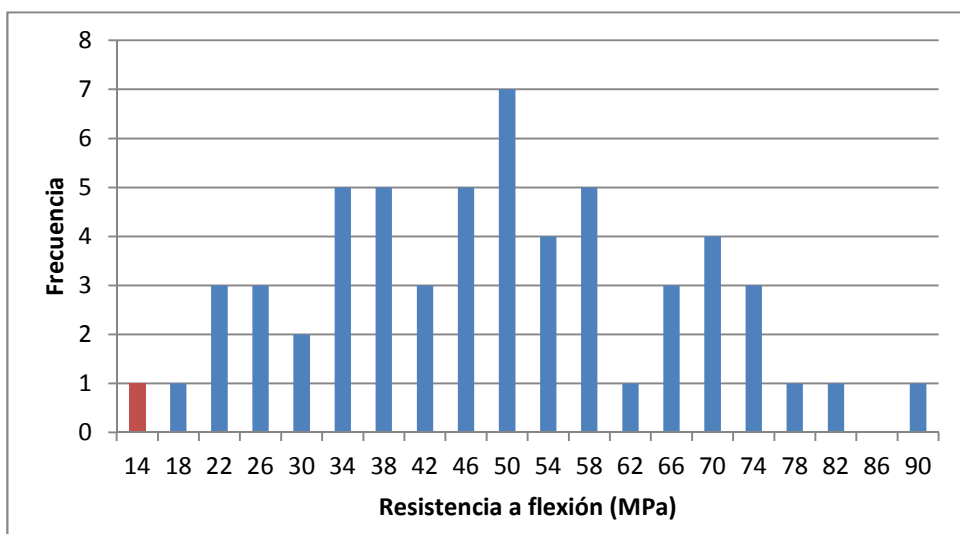
Gráfico B22. Histograma de resistencia a flexión para el muestreo del Litoral clasificado.
