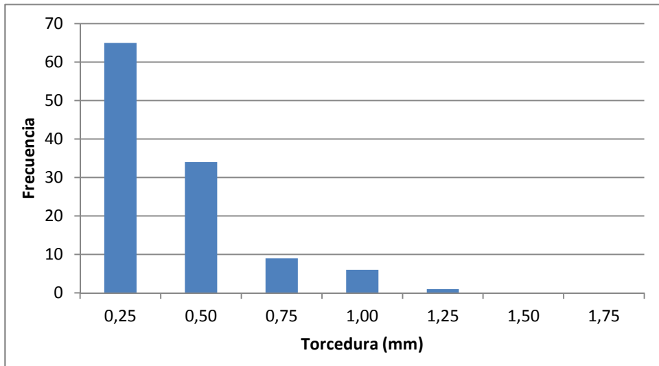
Gráfico B8. Histograma de frecuencia de torcedura para el muestreo de procedencia del Suroeste.
