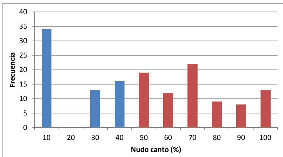
Gráfico B17. Histograma de frecuencia de nudo canto para el muestreo de procedencia del Suroeste.
