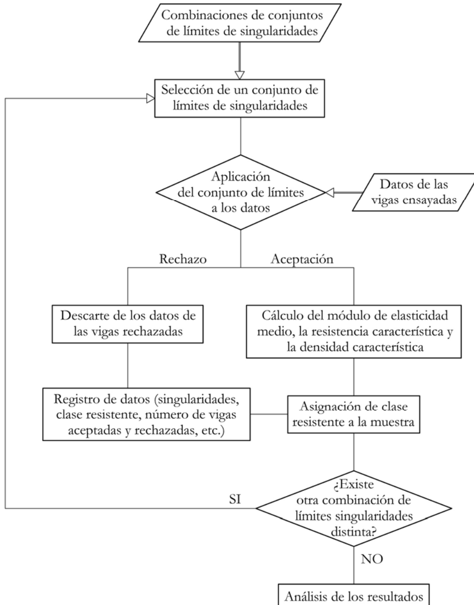
Figura 6. Diagrama de flujo del script.
