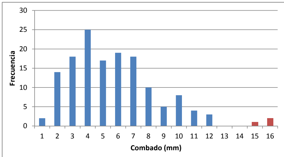
Gráfico B2. Histograma de frecuencia de combado para el muestreo de procedencia del Suroeste.
