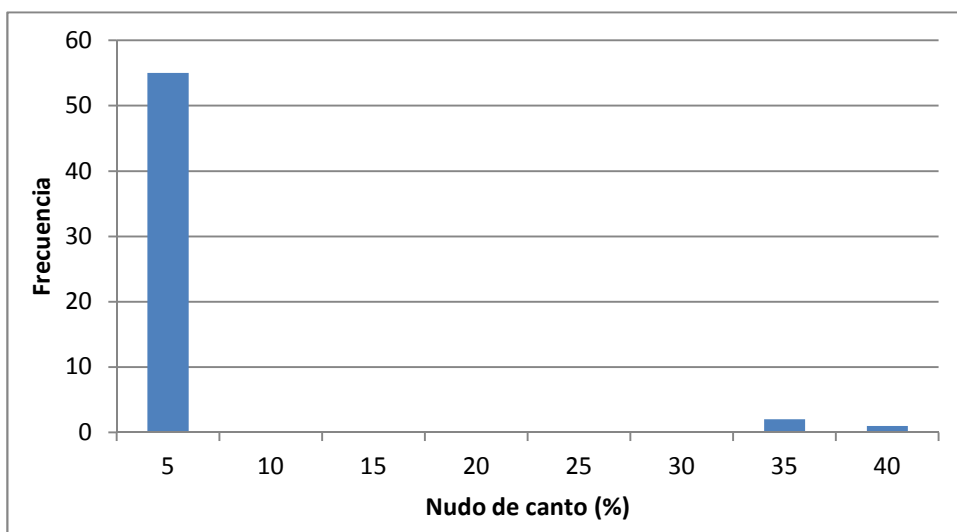
Gráfico B40. Histograma de nudo de canto para el muestreo del Litoral clasificado.
