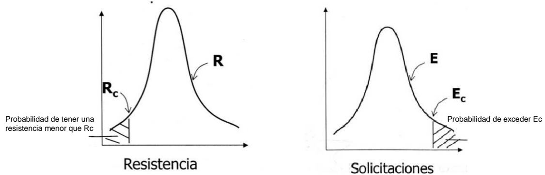
Figura 1.4. Distribución gaussiana de valores de a) resistencias y b) efectos de cargas
