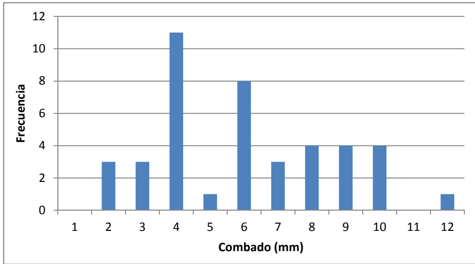
Gráfico B29. Histograma de combado para el muestreo del Suroeste clasificado.
