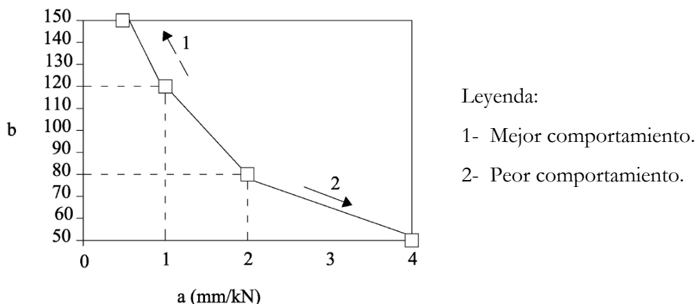
Figura 1 – Rango recomendado en la EN 1995-1-1 de los valores de a y b y de la relación entre sí.
