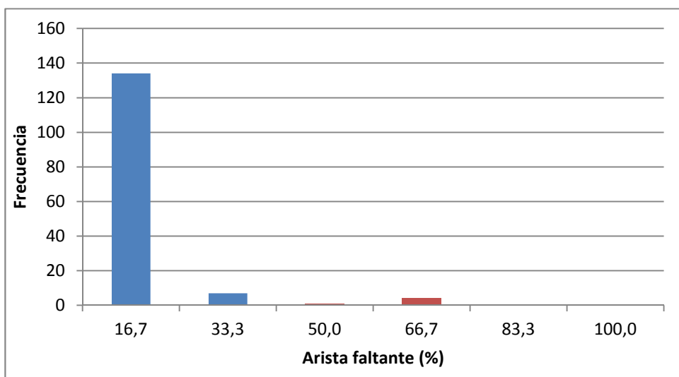
Gráfico B11. Histograma de frecuencia de arista faltante para el muestreo de procedencia del Suroeste.
