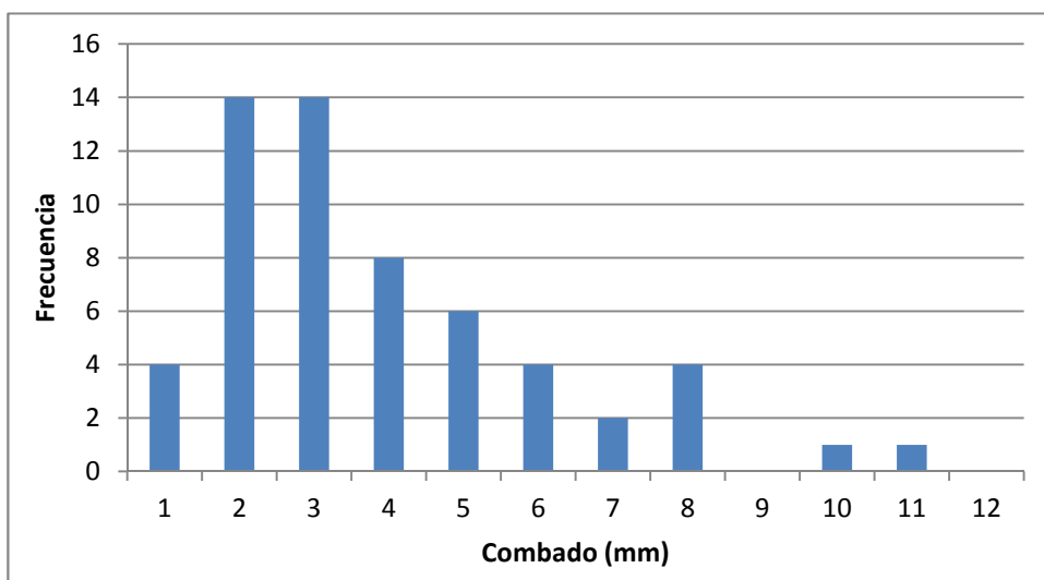
Gráfico B28. Histograma de combado para el muestreo del Litoral clasificado.
