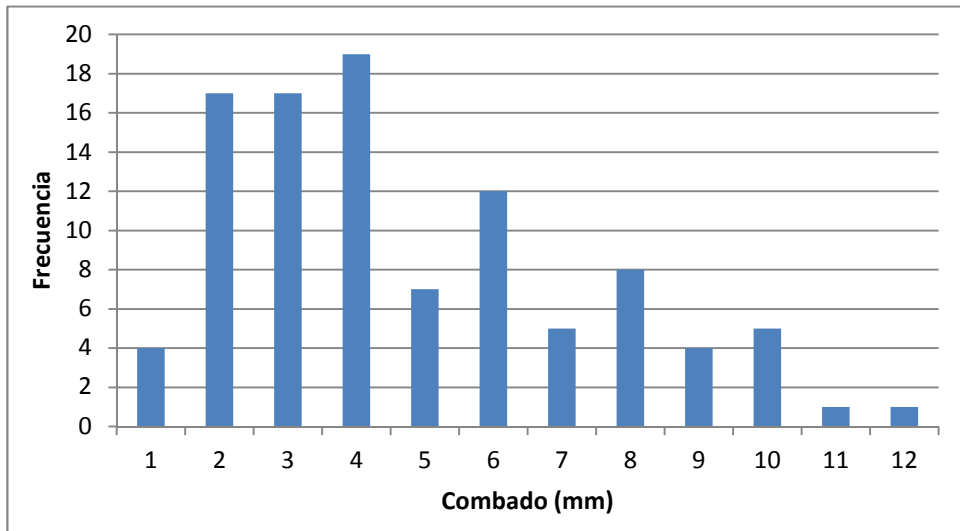
Gráfico B30. Histograma de combado para todas las vigas clasificadas.
