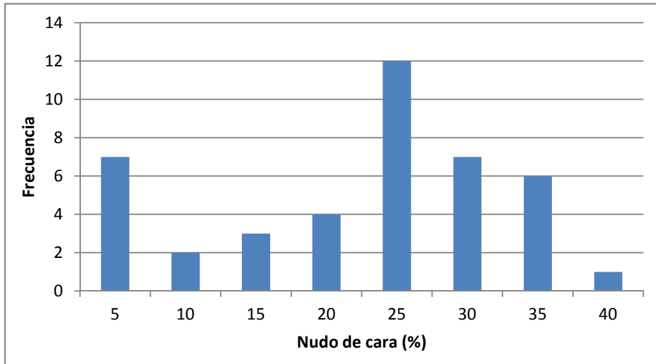
Gráfico B39. Histograma de nudo de cara para todas las vigas clasificadas.
