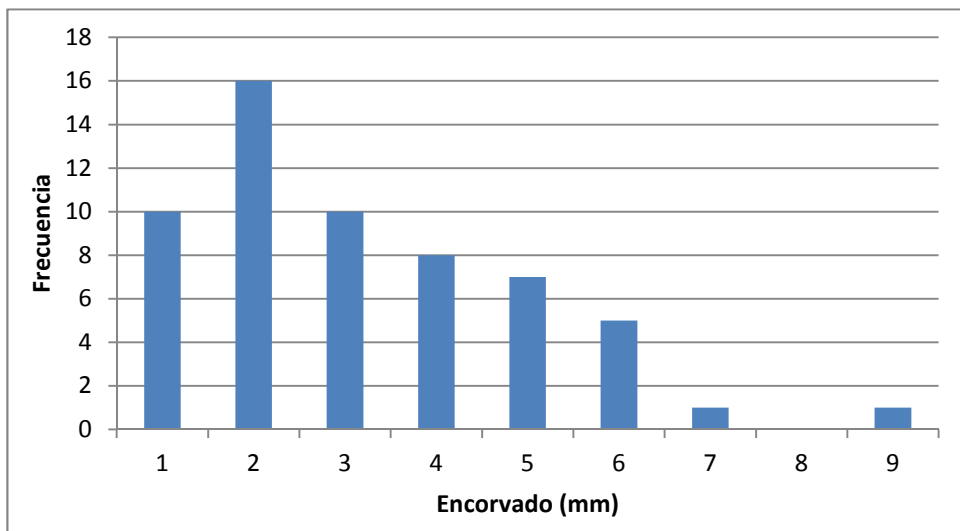
Gráfico B31. Histograma de encorvado para el muestreo del Litoral clasificado.
