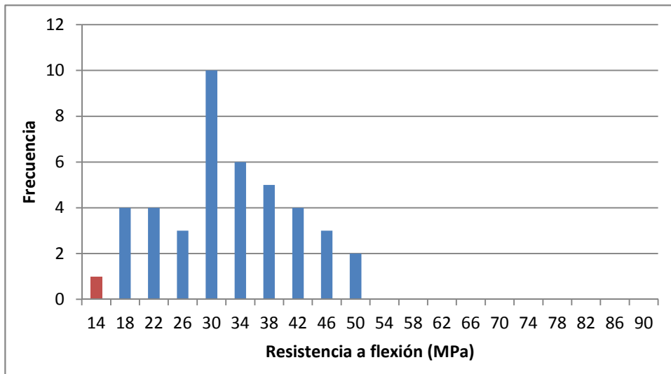
Gráfico B23. Histograma de resistencia a flexión para el muestreo del Suroeste clasificado.
