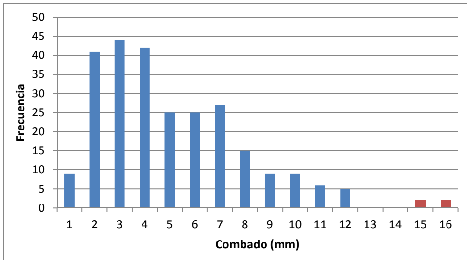
Gráfico B4. Histograma de frecuencia de encorvado para el muestreo de procedencia del Litoral.
