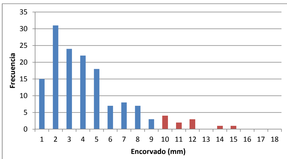
Gráfico B5. Histograma de frecuencia de encorvado para el muestreo de procedencia del Suroeste.
