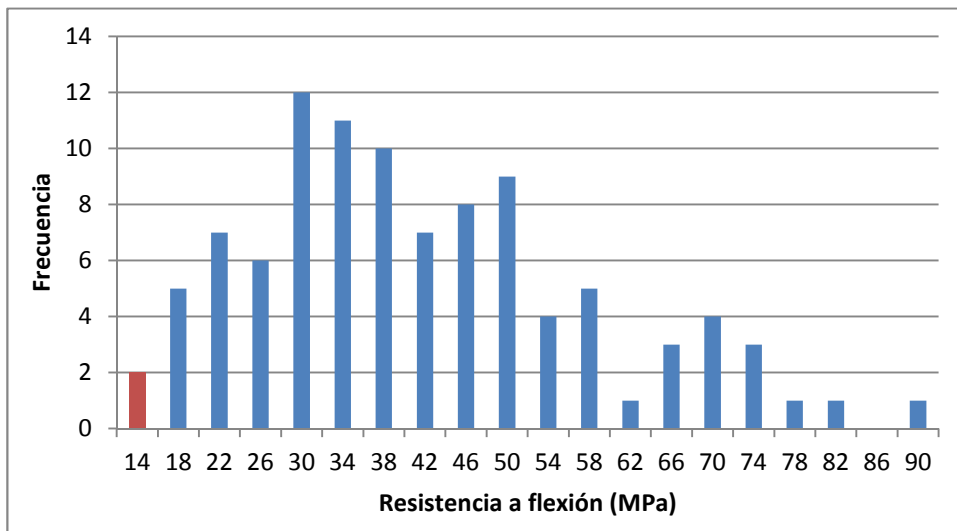
Gráfico B24. Histograma de resistencia a flexión para todas las vigas clasificadas.
