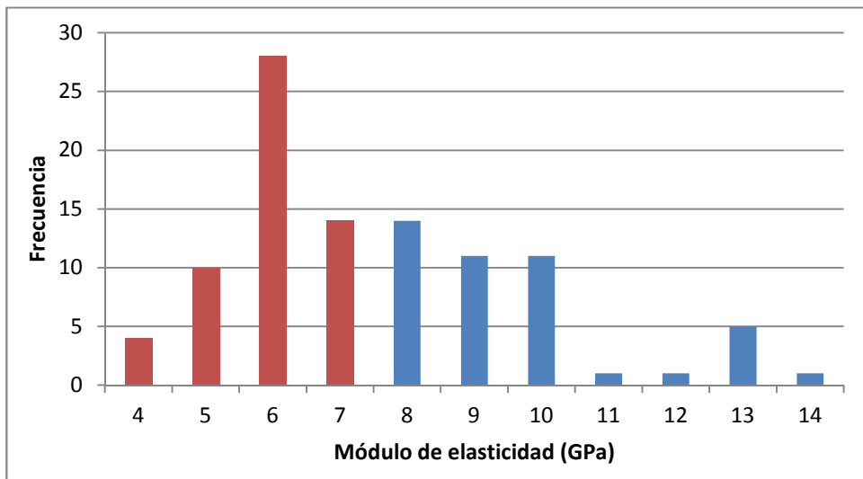
Gráfico B21. Histograma de módulo de elasticidad para todas las vigas clasificadas.
