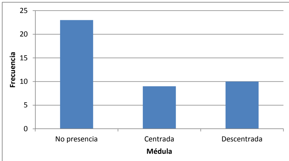
Gráfico B26. Histograma de presencia de médula para el muestreo del Suroeste clasificado.
