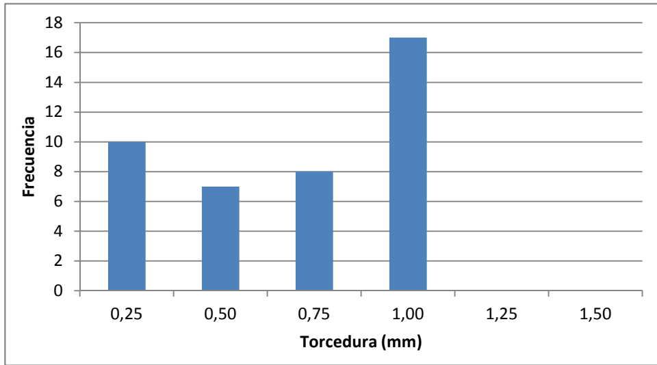
Gráfico B35. Histograma de torcedura para el muestreo del Suroeste clasificado.
