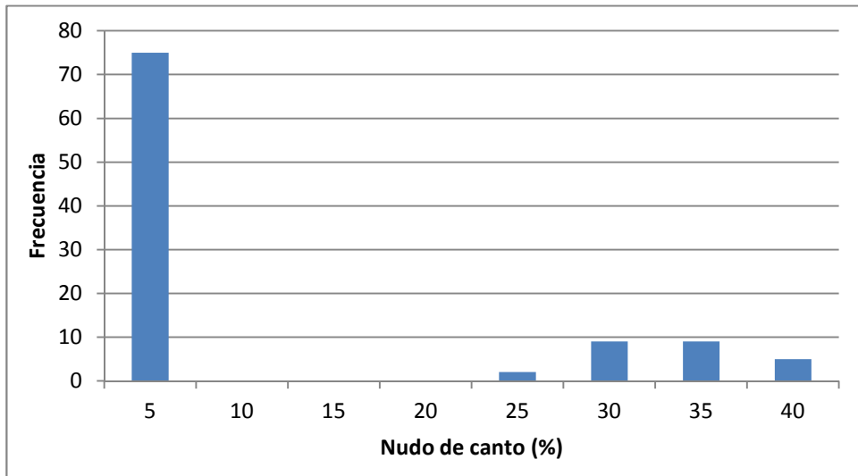
Gráfico B42. Histograma de nudo de canto para todas las vigas clasificadas.
