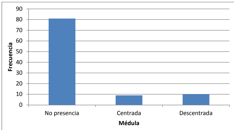
Gráfico B27. Histograma de presencia de médula para todas las vigas clasificadas.
