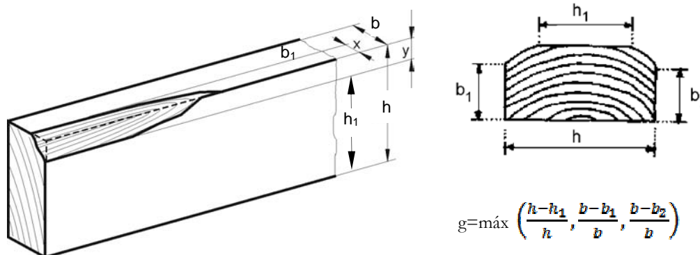
Figura 5. Arista faltante o gema
